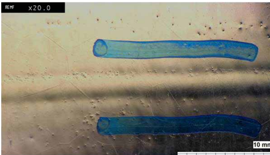
B16; 0,8mm; 4–8 \mu\text{m} Zinnschichtdicke; SnPUR
