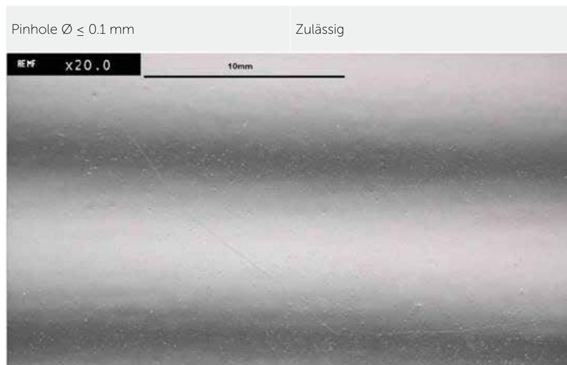
CuNiSi, C19010; 0,32 mm Materialdicke, 3–6µm Sn
