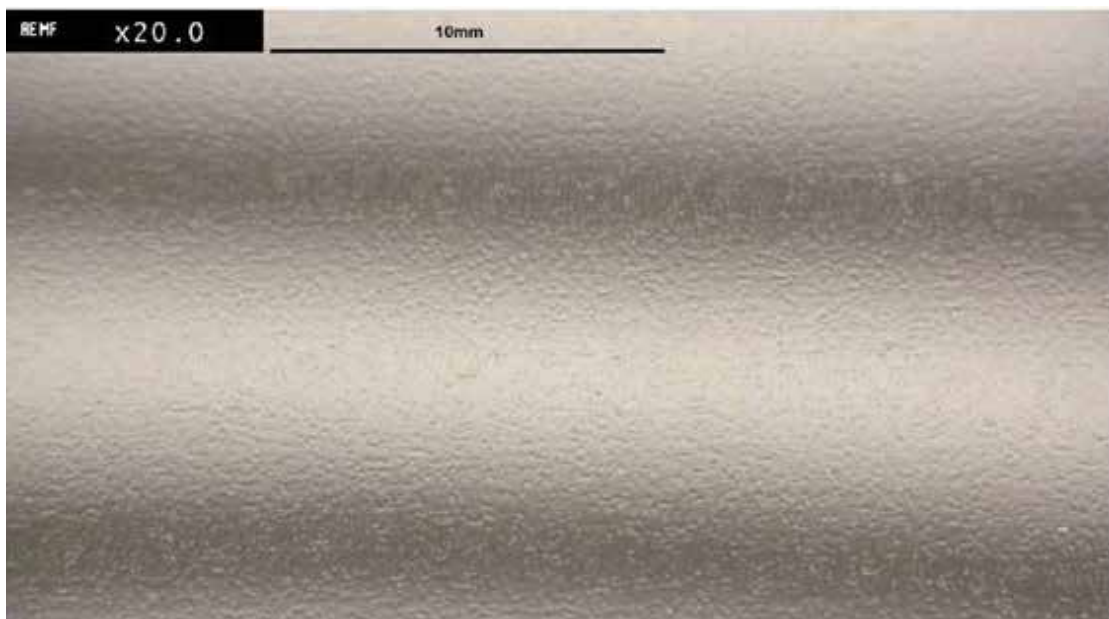
CuNiSi, C19010, 0,2 mm Materialdicke, 1–2 \mu\text{m} Sn
