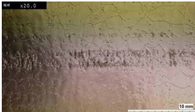
M38; 0,8mm; 2–4µm Zinnschichtdicke; SnPUR
