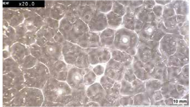
M30; 0,342mm; 3–5 \mu\text{m} Zinnschichtdicke; SnPUR
