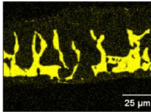
Verteilung Phosphor
