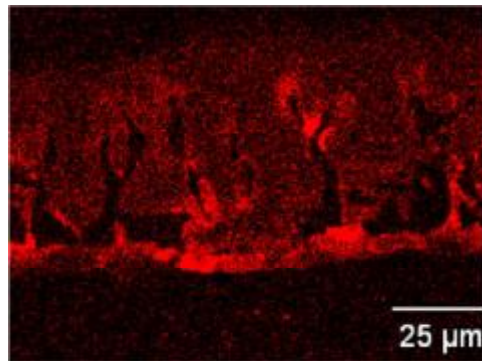
Verteilung Silber
