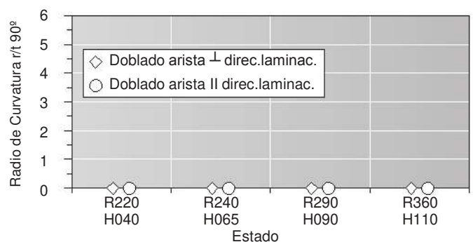
Doblado (Espesor de la cinta t ≤ 0.5 mm)
