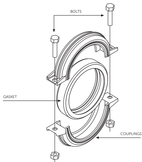
Fig. 14.3 VICTAULIC® CONNECTION
